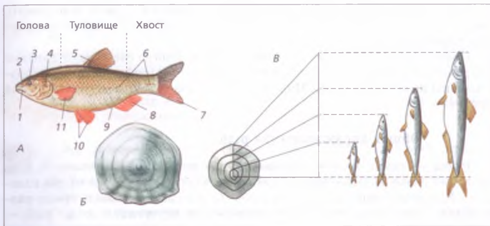
Рис. 112. Внешнее строение рыбы: А — общий план строения: 1 — рот; 2 — ноздря; 3 — глаз; 4 — жаберная крышка; 5 — спинной плавник; 6 — боковая линия; 7 — хвостовой плавник; 8 — анальный плавник; 9 — анальное отверстие; 10 — брюшные плавники; 11 — грудной плавник; Б — чешуя с годовыми кольцами; В — определение возраста рыбы
